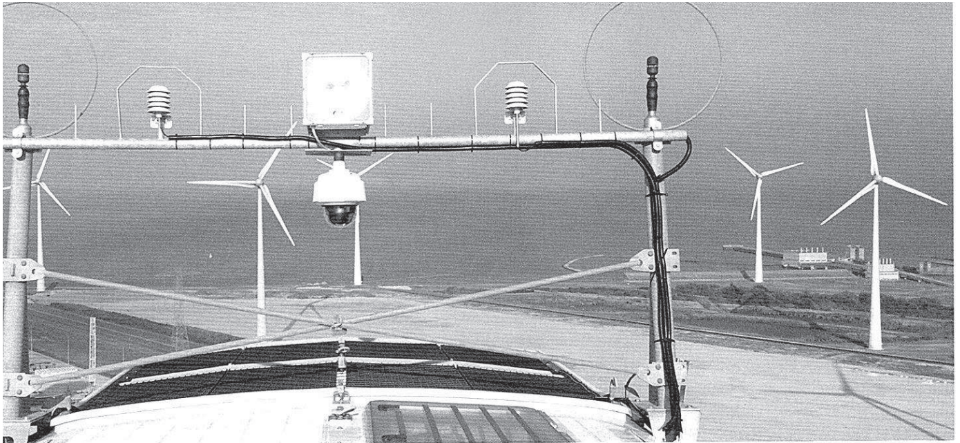
Frühwarnanlage: Die Hamburger Firma Leine & Linde hat ein Sensorsystem entwickelt, das Meldung macht, wenn die Wetterbedingungen am Windrad so sind, dass sich mit hoher Wahrscheinlichkeit Eis auf den Flügeln bilden wird.
