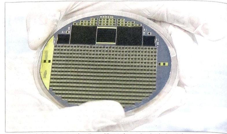
Wafer mit Vierfach-Konzentratorsolarzellen und Teststrukturen: Forscher des Fraunhofer-Instituts für Solare Energiesysteme in Freiburg erreichen inzwischen im Labor einen Wirkungsgrad von 43,6 %. Foto: Fraunhofer ISE
