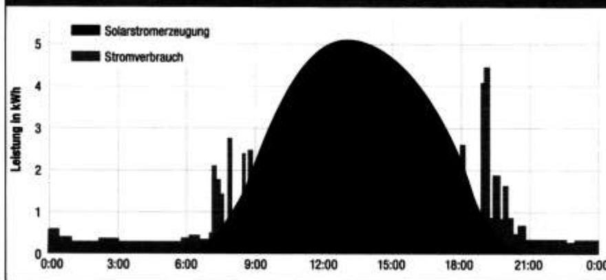
Abb. 1: Anzeige Solarstromerzeugung und Eigenverbrauch bei der VisionBox von Conergy (Beispiel für einen schönen Sommertag)
