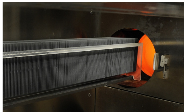
Schlüsselprozess: Durch Phosphordiffusion, das Einbringen von Phosphoratomen in den Halbleiter, wird die Solarzelle elektrisch leitfähig. Die Öfen für dieses Verfahren stammen vorwiegend aus Deutschland. (Foto: Solarworld)
